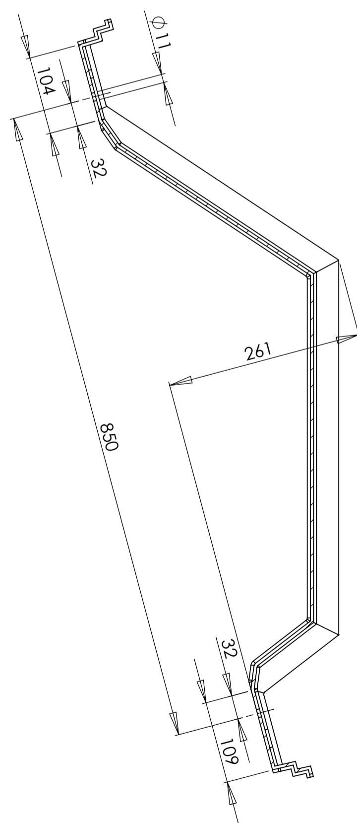
ŘEZ B-B MĚŘITKO 1 : 5
