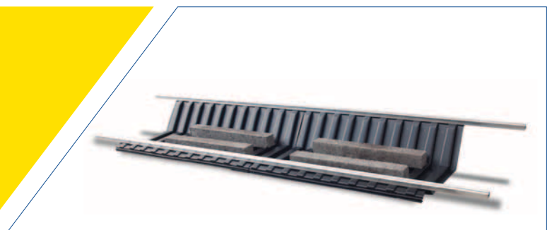
Aufbau VarioTwin Large 15° mit horizontaler Profilanordnung
